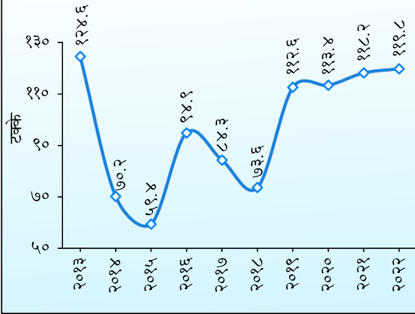
आलेख ७.२ : राज्यात पडलेल्या पावसाची सरासरी पावसाशी टक्केवारी (दशकातील)
